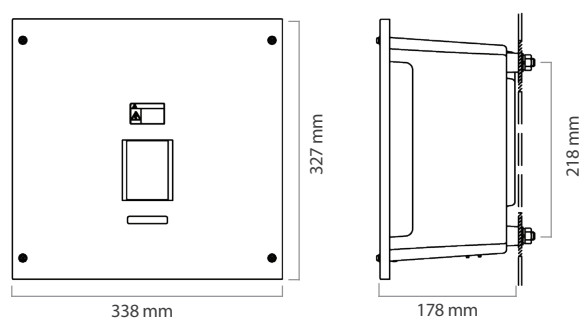
整合筐 NQD-2597/2598 質量: 約0.87 kg NQD-2597 約0.76 kg NQD-2598
