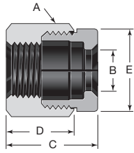
Innengewinde
